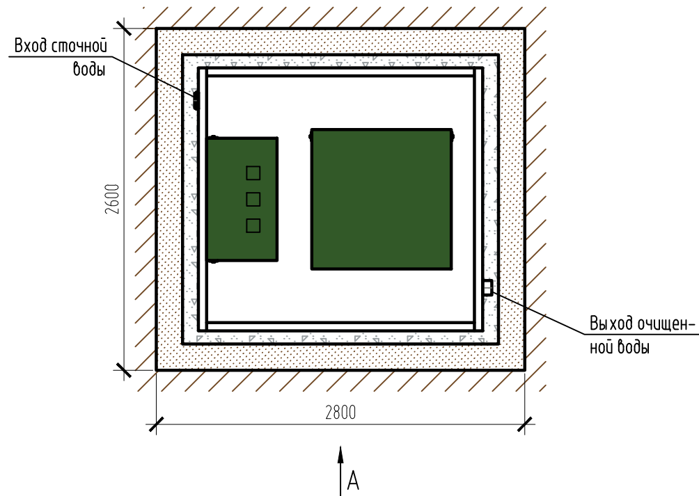
Вид сверху
